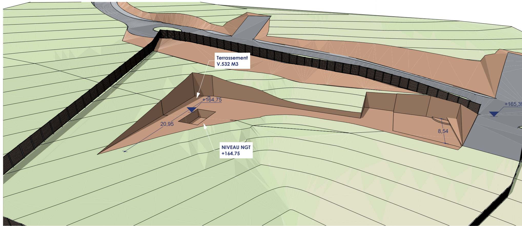
OP-3D18 L52_Terrassement 1:200
