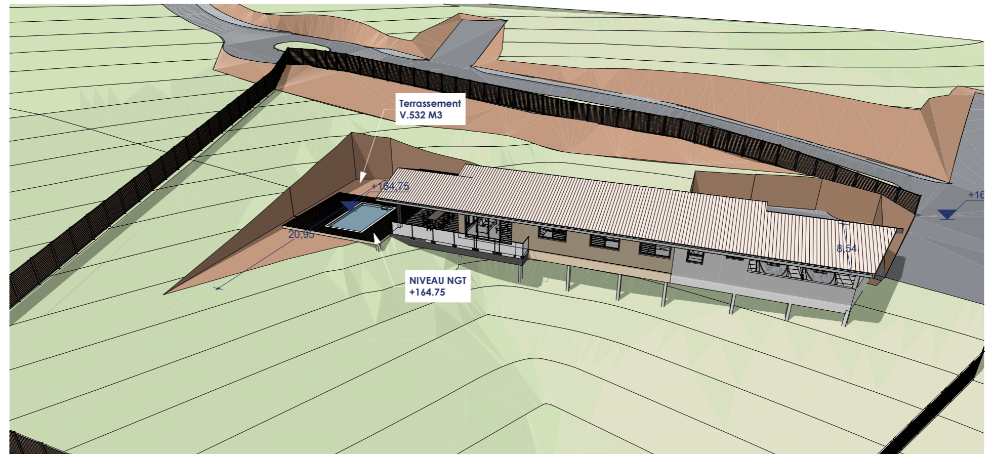
OP-3D18 L52_Terrassement avec Maison 1:200
