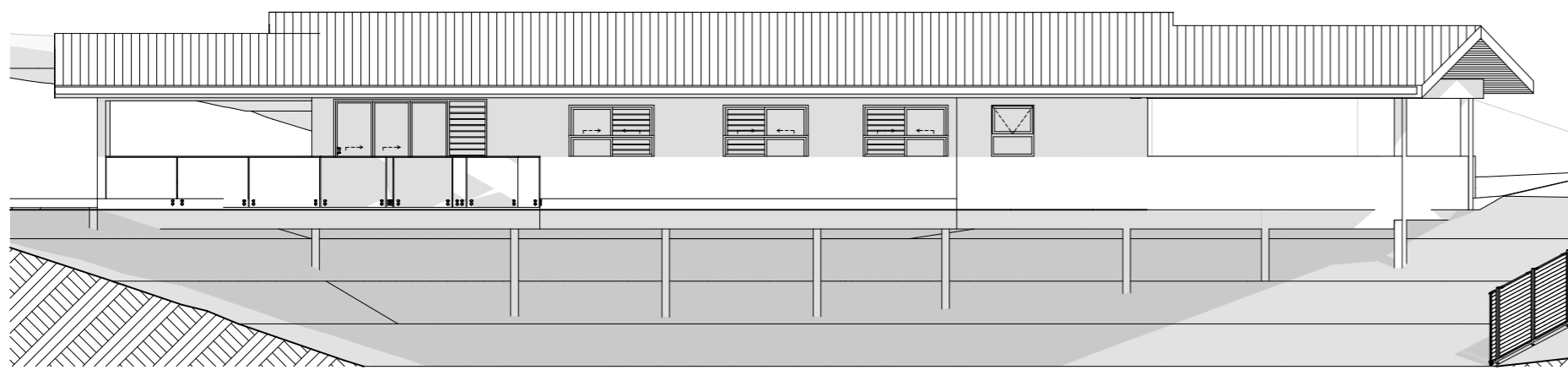
SE Façade Sud Est 1:150
