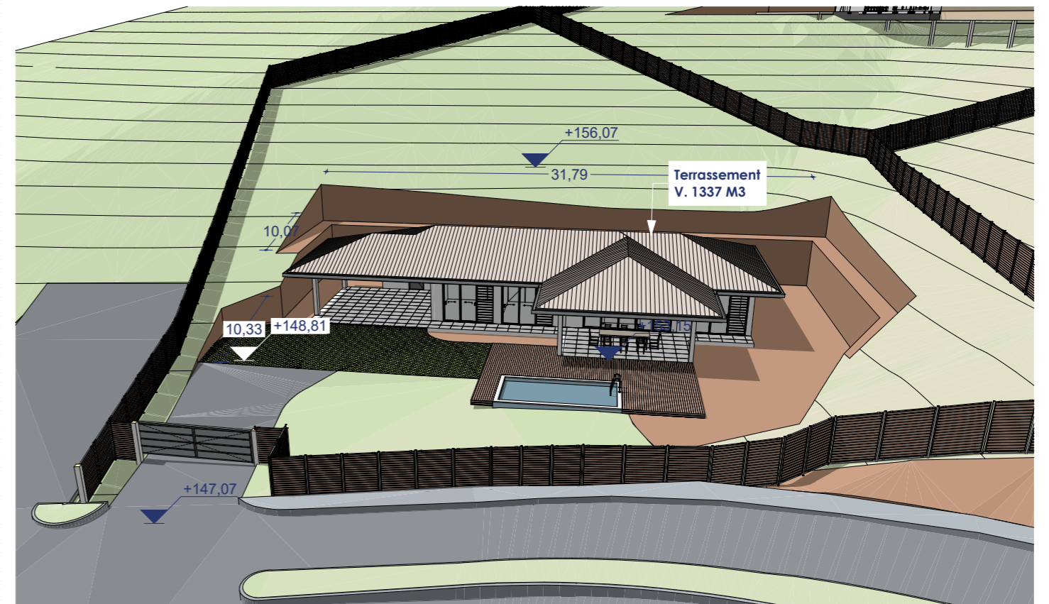
Perspective L44, Perspective L44 Avec maison
